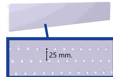
PERFORIERTE RÜCKWAND (M.2)
